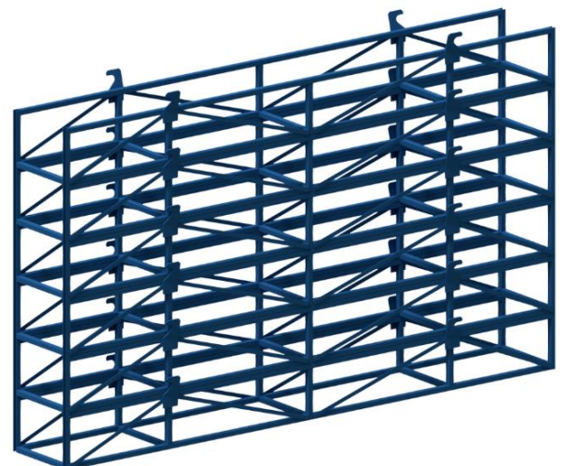
LP mit offenen Einhakblechen – kompatibel mit Kranhubzangen
